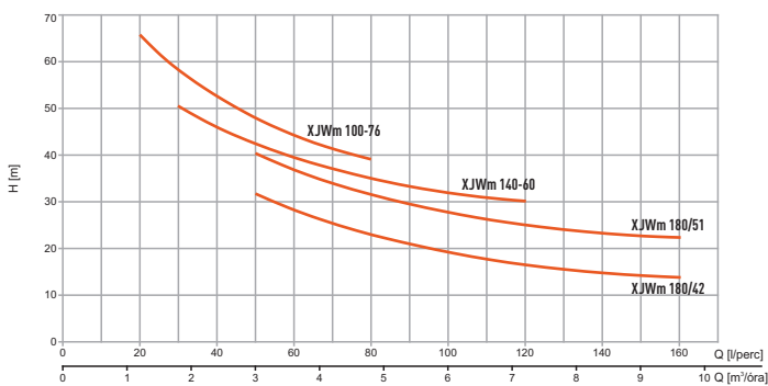
Teljesítmény-diagram
