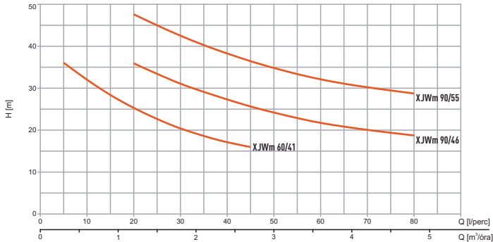
Teljesítmény-diagram
