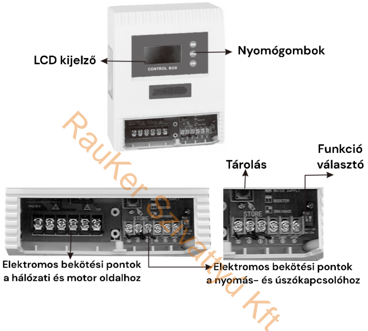
LCD kijelző
